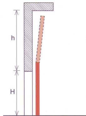
درب سکشنال نوع V (عمودی) بازشوی عمودی
