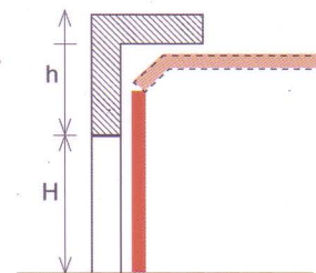
درب سکشنال نوع R بازشوی افقی در حداقل فضا
