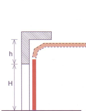
درب سکشنال نوع N (متداول) بازشوی افقی
