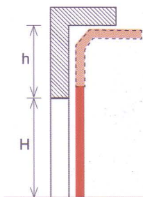
درب سکشنال نوع S (نیمه افقی) بازشوی نیمه عمودی - افقی
